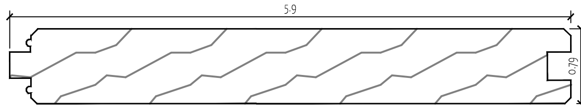
1x6 CLADDING - T/G (JEM)
