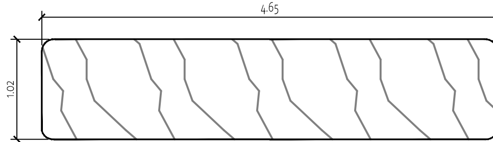
5/4 X 5 DECKING - PaCS - D4 NO GROOVE (JEM)
